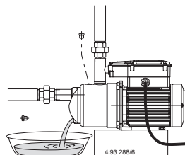
Fig. 5 Scarico Draining Entleerung Vidange Vaciado Avtappning Aftappen Αποστράγγιση Слив 排空
