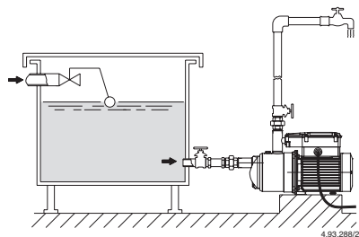
Fig. 1 Funzionamento sotto battente Positive stion head operation Zulaufbetrieb Fonctionnement en charge Funcionamiento bajo carga Tillrinning sugsidan Toeloopsituatie Θέση λειτουργίας με θετική αναρρόφηση Работа под гидравлическим напором 正压上水头的操作
